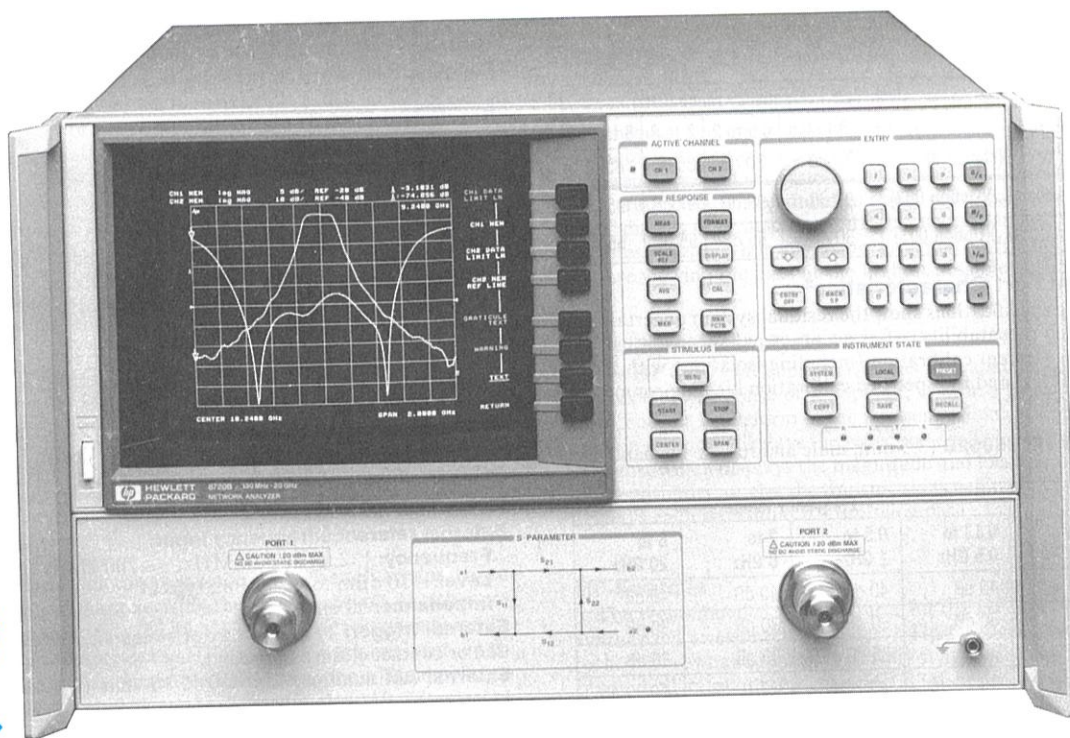
HP 8720B
